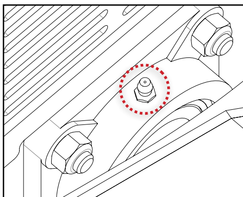
Roulement d'arbre de volant avant
