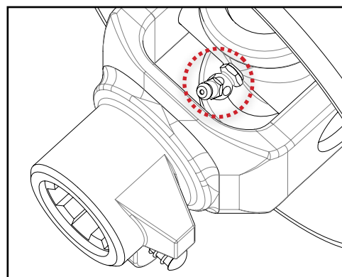
Joint en U d'arbre de prise de force 2
