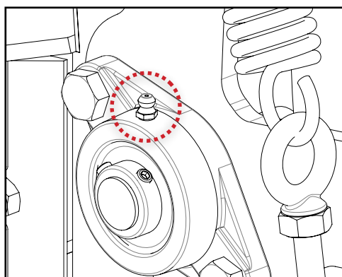
Roulement du rouleau d'alimentation
